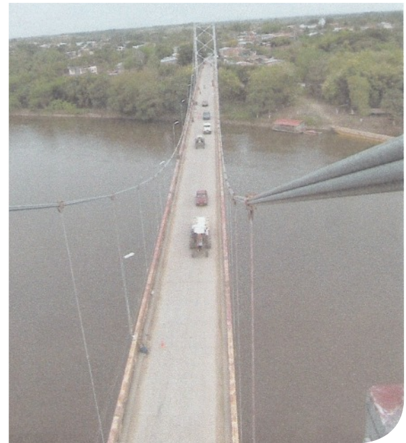
PUENTE RAMON NONATO PEREZ LUZ = 50 METROS CLIENTE: INVIAS
